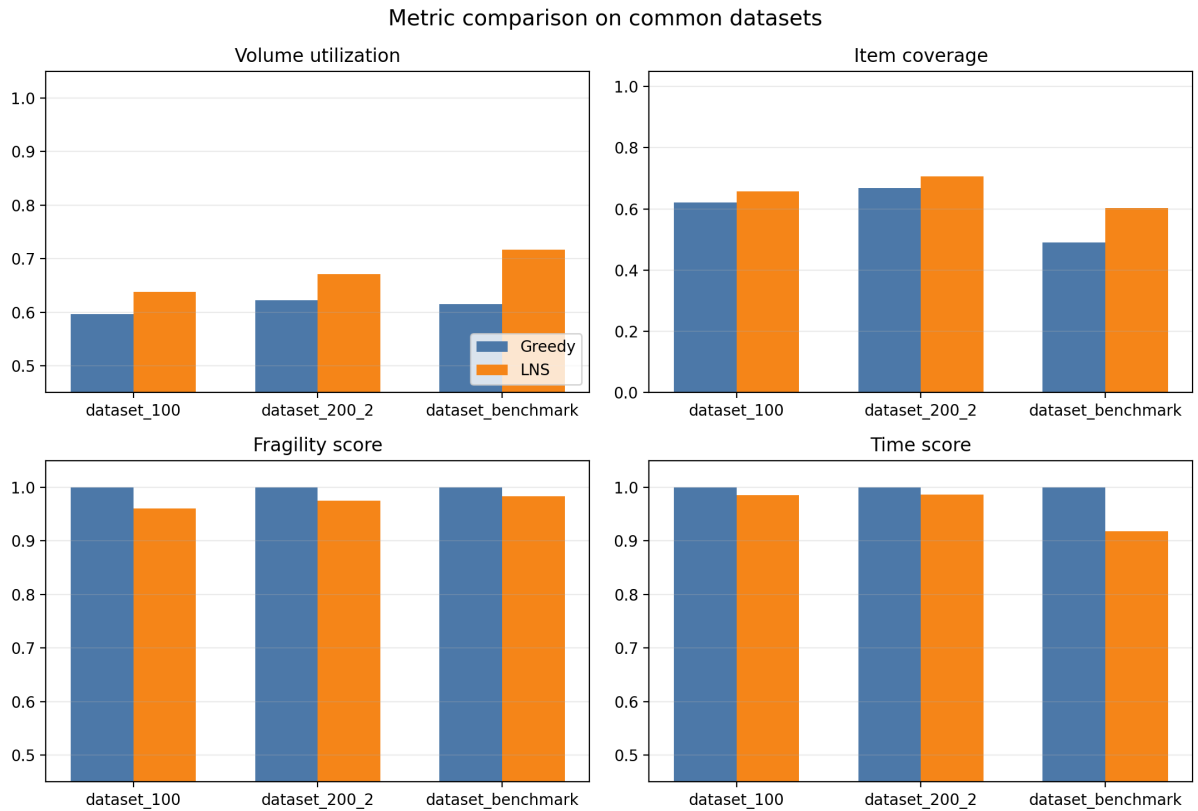
Рис. 8. Сравнение компонент метрики для LNS и greedy
